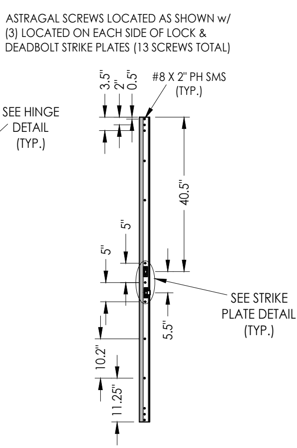
ASTRAGAL
