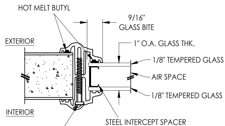
1/2 LITE
