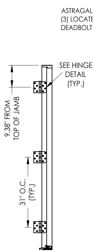
HINGE JAMB
