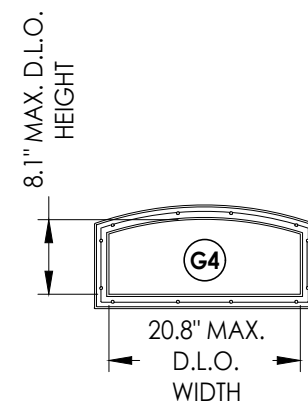
CAMBER TOP
